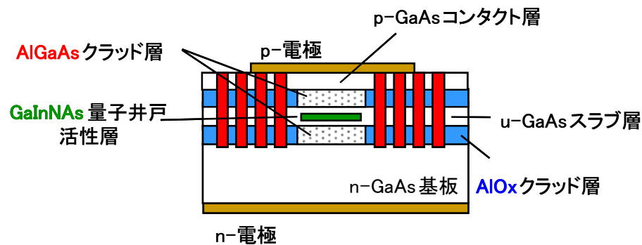
開発するレーザの構造（俯瞰図および断面図）
