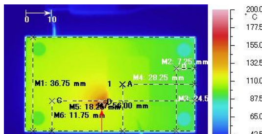
SiCパワーデバイスの高温動作と モジュール温度分布解析
