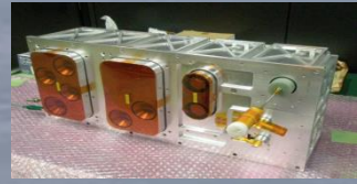
宇宙ステーション搭載雷観測センサ
