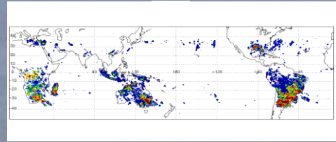
人工衛星より観測した雷活動頻度分布
