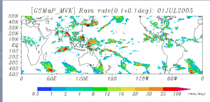
高精度高分解能全球降水マップ
